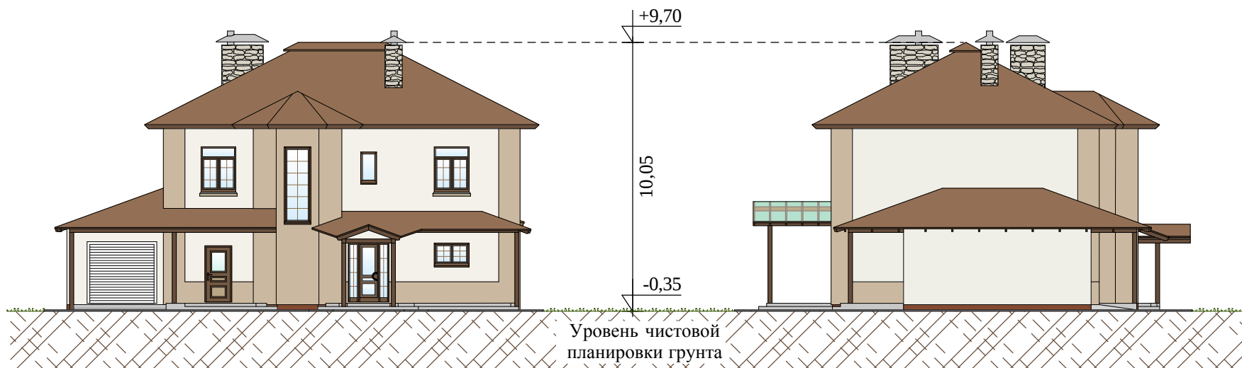
Вид фасада спереди
